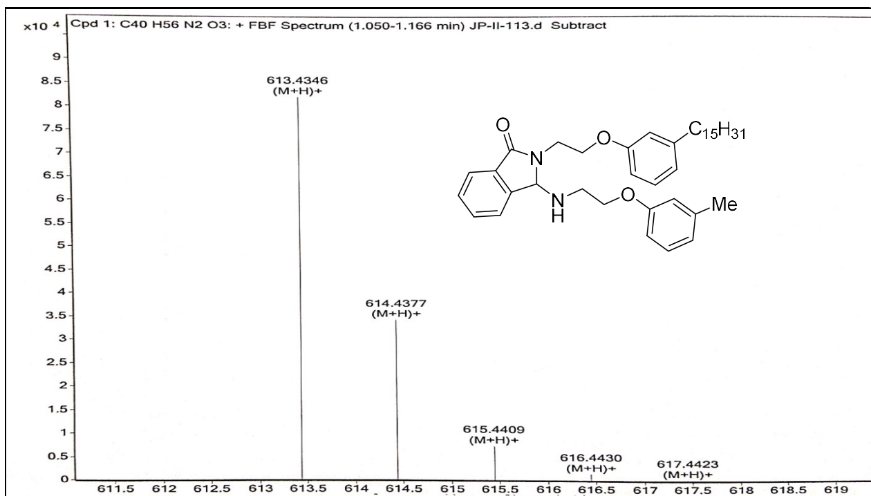
HRMS spectrum of 2-(2-(3-pentadecylphenoxy)ethyl)-3-((2-( m -tolylloxy)ethyl)amino)isoindolin-1-one 3c .
