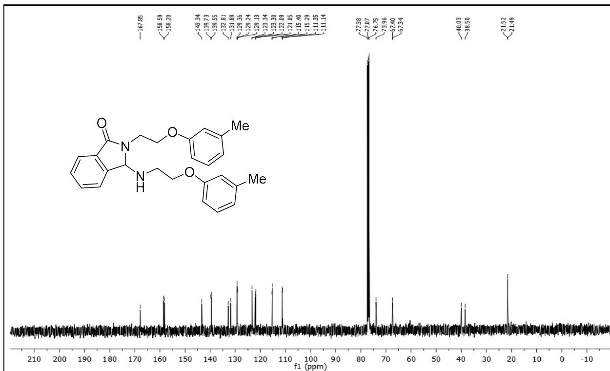
13 C NMR (100 MHz, CDCl 3 ) spectrum of 2-(2-( m -tolyloxy)ethyl)-3-((2-( m -tolyloxy)ethyl)amino)isoindolin-1-one 3d .
