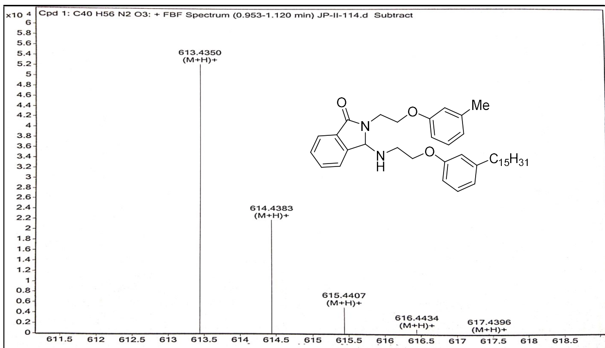
HRMS spectrum of 3-((2-(3-pentadecylphenoxy)ethyl)amino)-2-(2-( m -tolylxy)ethyl)isoindolin-1-one 3b .
