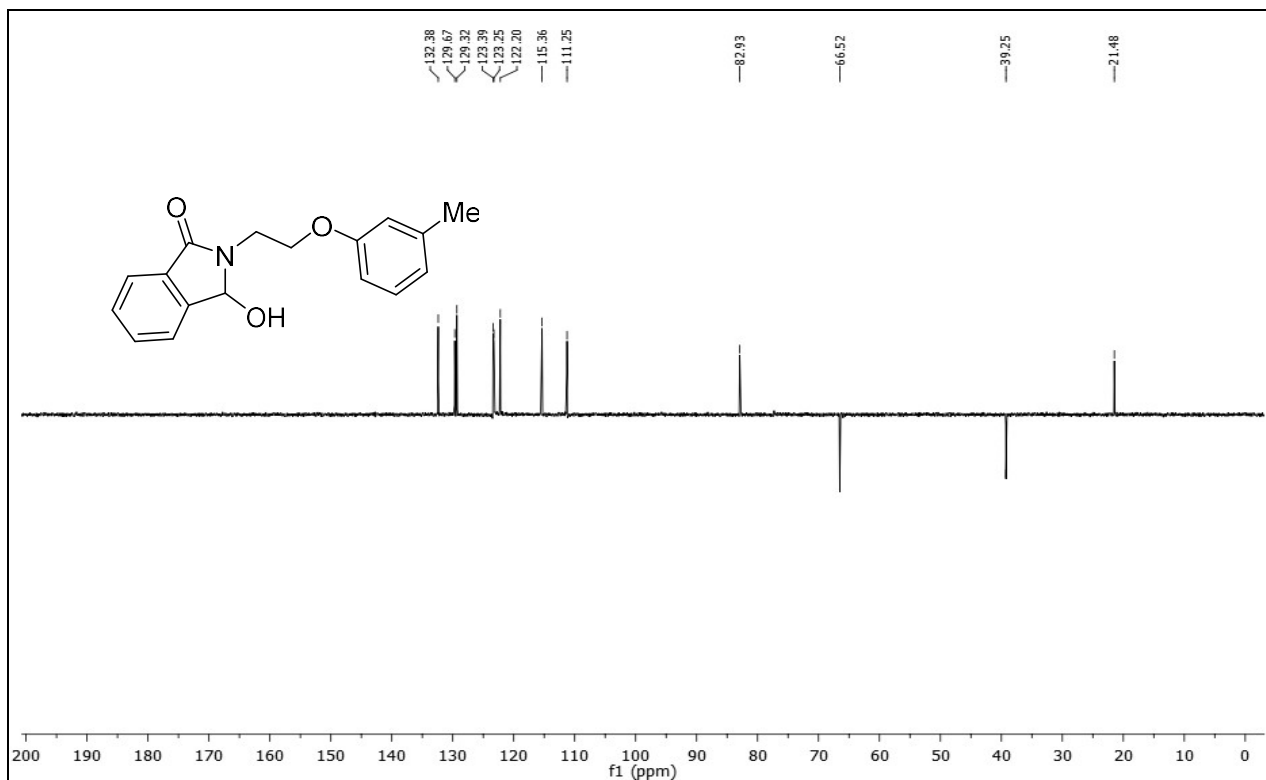
DEPT-135 spectrum of 3-hydroxy-2-(2-( m -tolylloxy)ethyl)isoindolin-1-one 7b .
