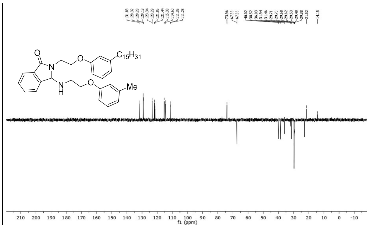
DEPT-135 spectrum of 2-(2-(3-pentadecylphenoxy)ethyl)-3-((2-( m -tolylloxy)ethyl)amino)isoindolin-1-one 3c .
