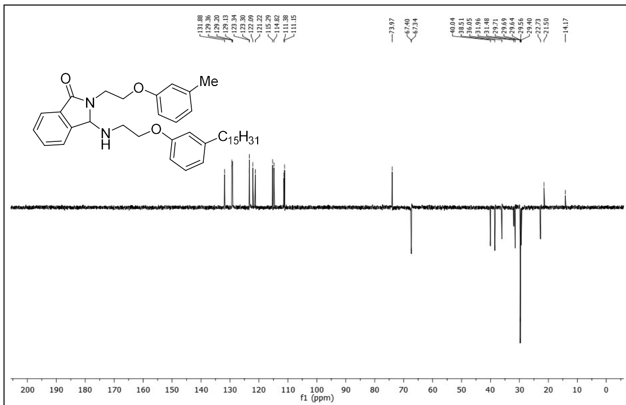
DEPT-135 spectrum of 3-((2-(3-pentadecylphenoxy)ethyl)amino)-2-(2-( m -tolylxy)ethyl)isoindolin-1-one 3b .
