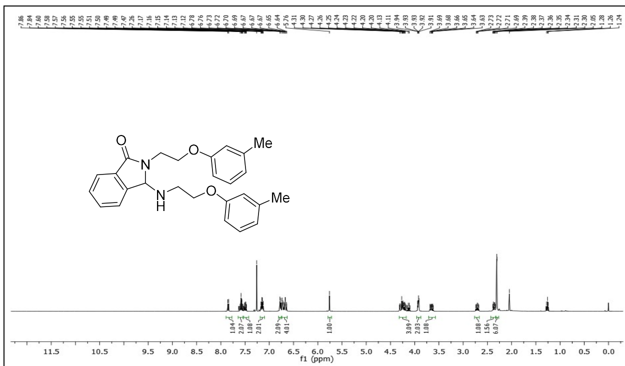
1 H NMR (400 MHz, CDCl 3 ) spectrum of 2-(2-( m -tolyloxy)ethyl)-3-((2-( m -tolyloxy)ethyl)amino)isoindolin-1-one 3d .
