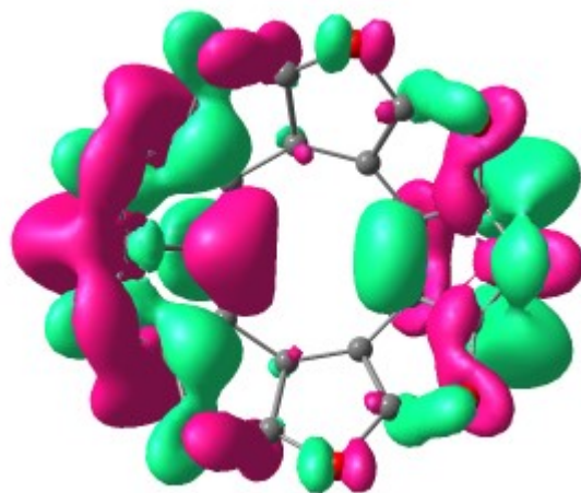
LUMO+2
