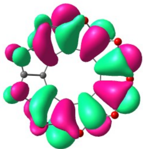
HOMO
