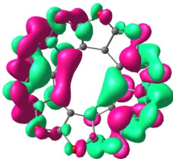
LUMO+2
