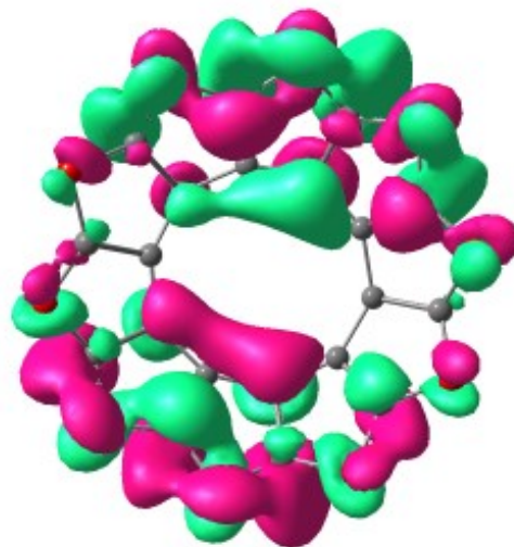
LUMO+2
