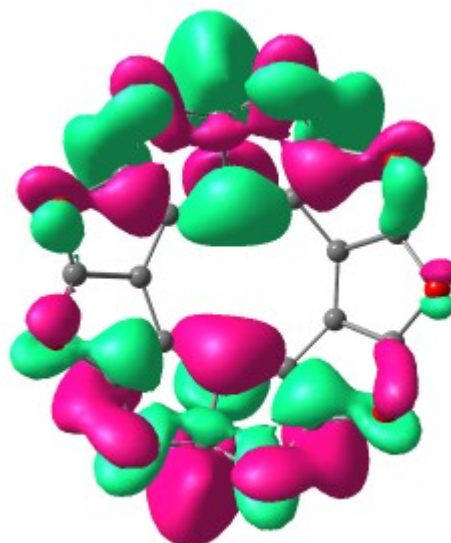
LUMO
