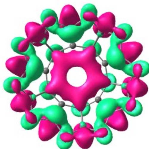
LUMO
