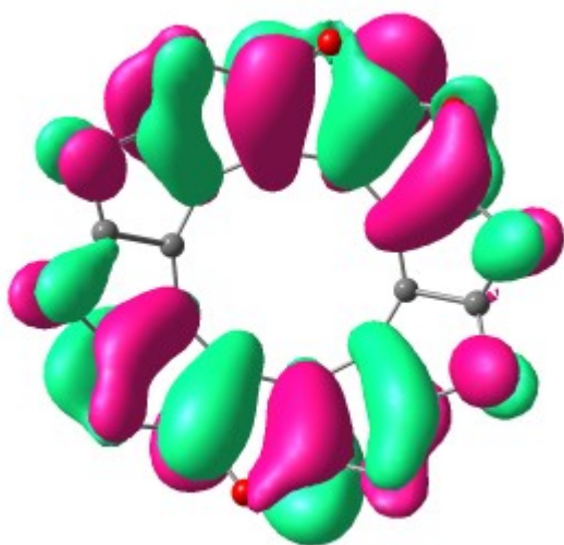
HOMO
