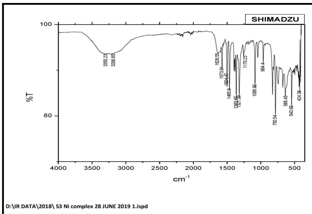
Fig. SI-4. IR spectrum of Ni(II) Complex
