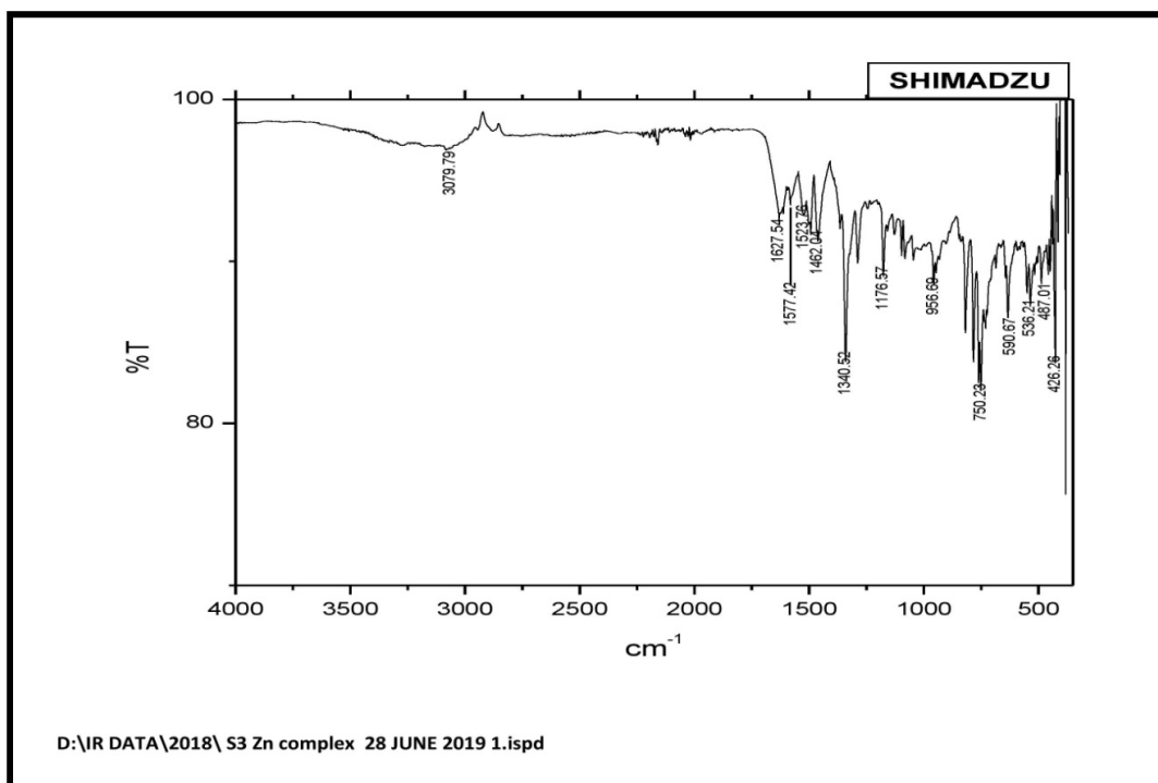
Fig. SI-6. IR spectrum of Zn(II) Complex
