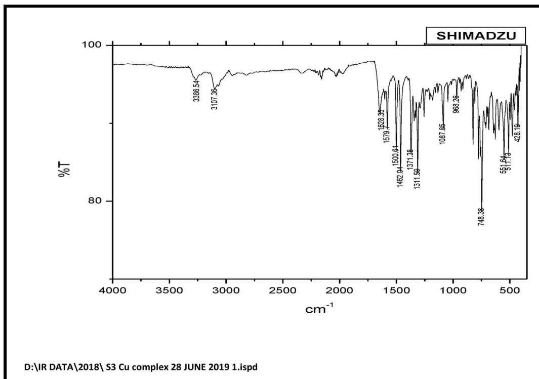
Fig. SI-5. IR spectrum of Cu(II) Complex
