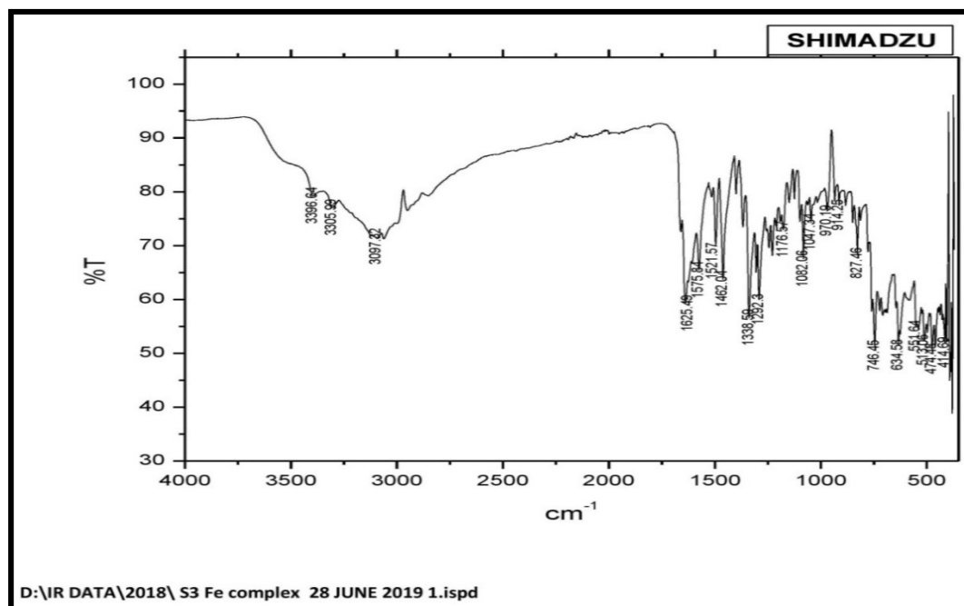
Fig. SI-2. IR spectrum of Fe(III) Complex
