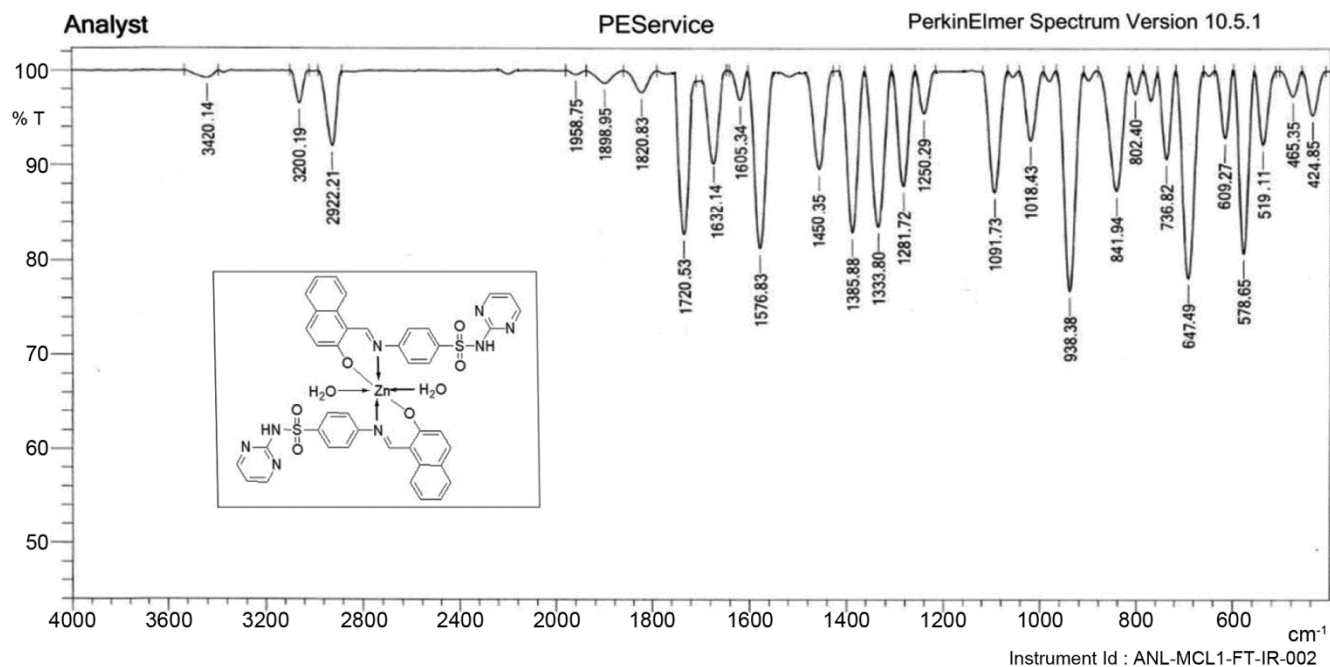
Suppl. Fig. S8 — IR spectrum of Zn Complex 5
