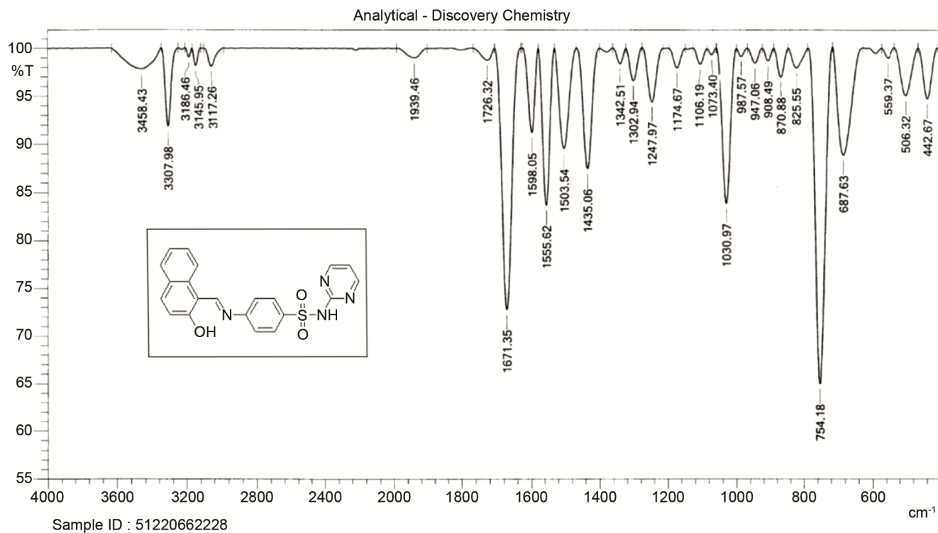
Suppl. Fig. S4 — IR spectrum of Ligand 3
